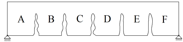
Рис. 1. До розрахунку комбінованих елементів за L \gg h
